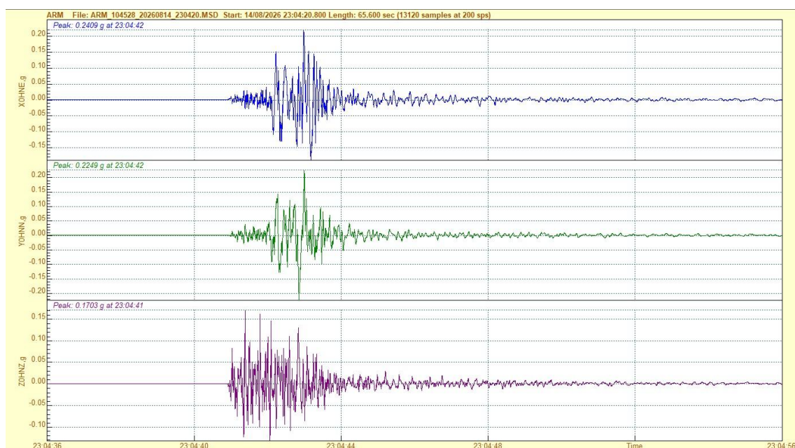
Figura 6. Acelerogramas registrados en la estación de Armilla correspondiente al terremoto de Mw 4,8 del 14/08/2026 23:04:40 (UTC).
